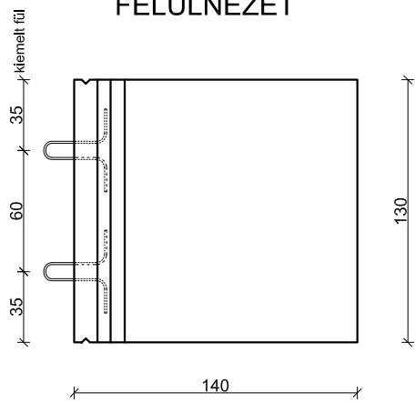
FELÜLNÉZET
